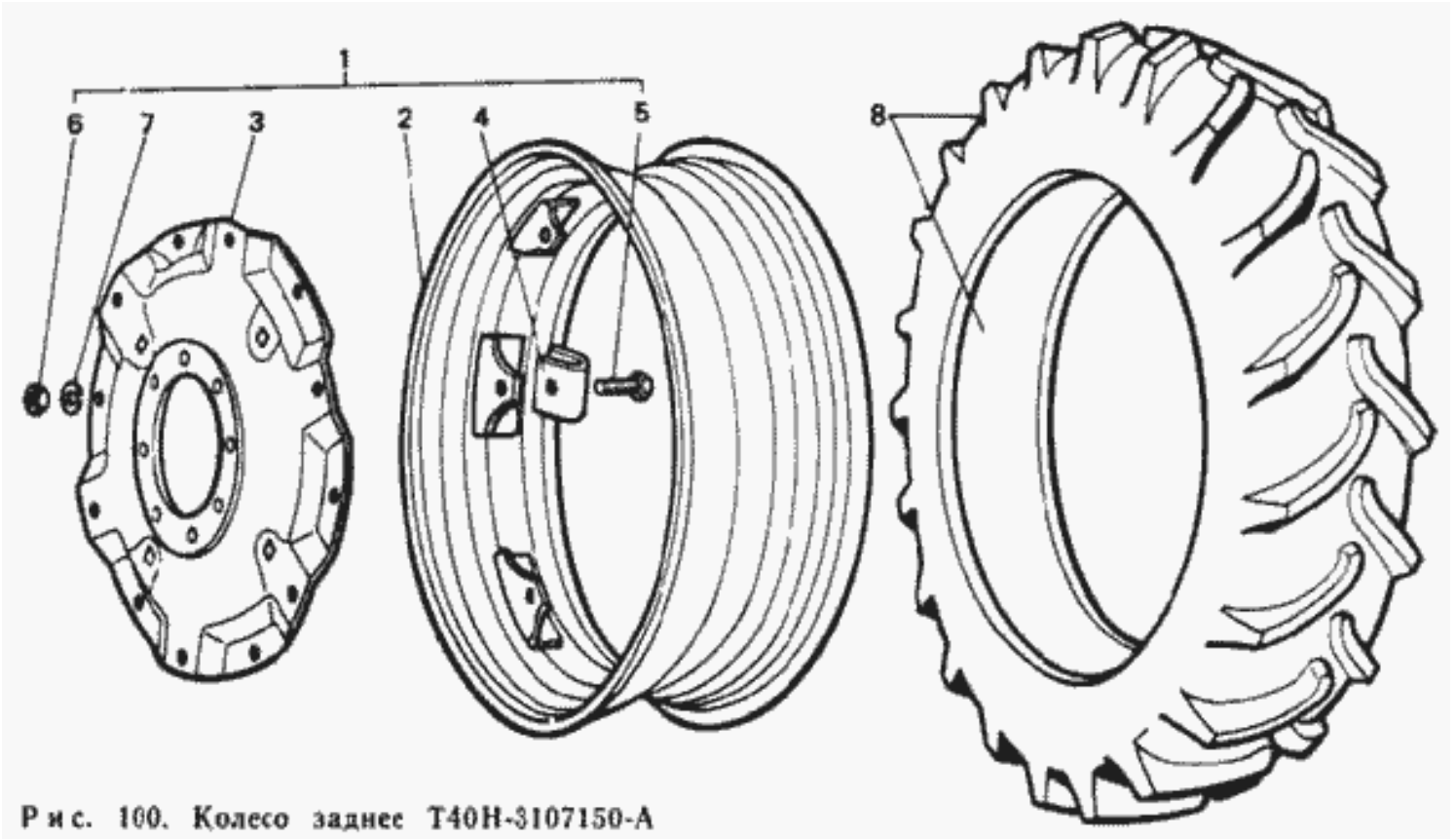
Рис. 100. Колесо заднее Т40Н-3107150-А.
